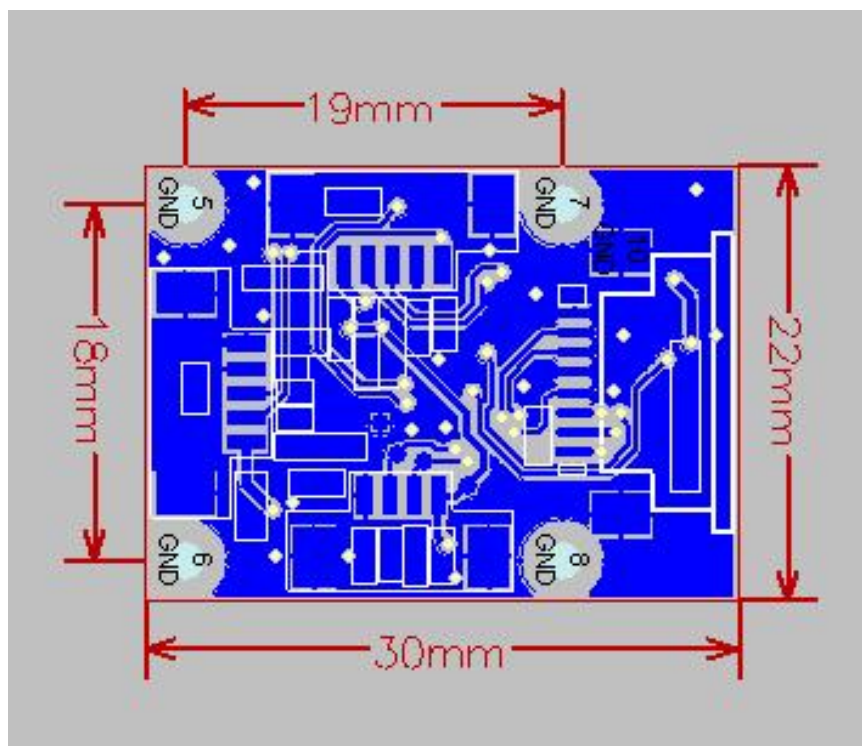
图2-2 AFM32主板尺寸图
