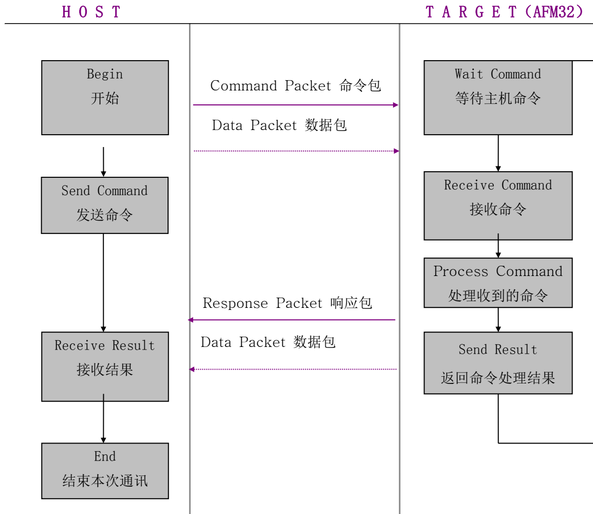
图4-1 通讯过程
