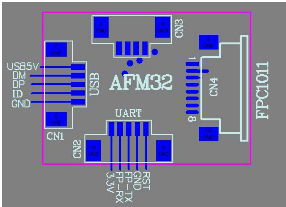
图2-4 AFM32接口定义图
