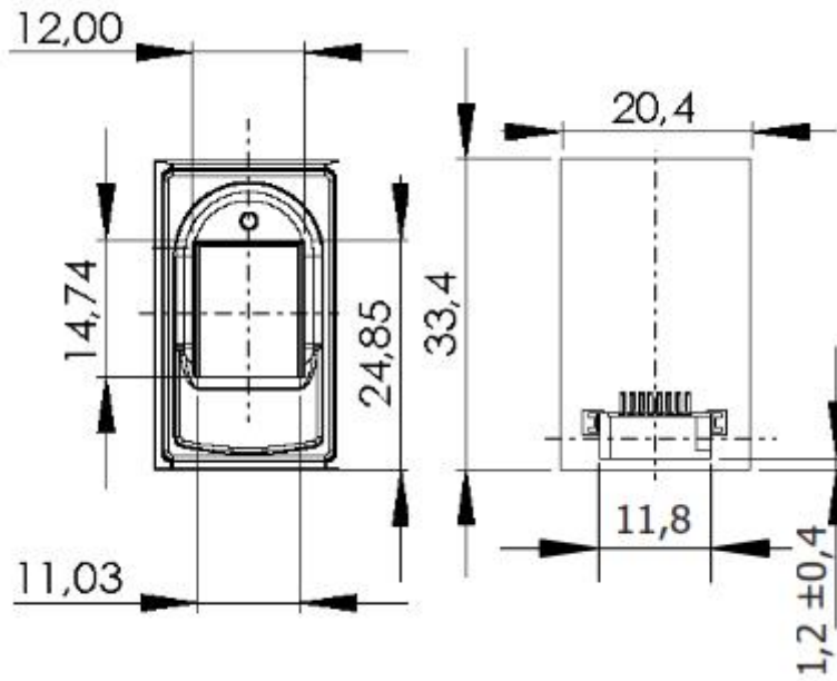
图2-3 FPC1011尺寸图
